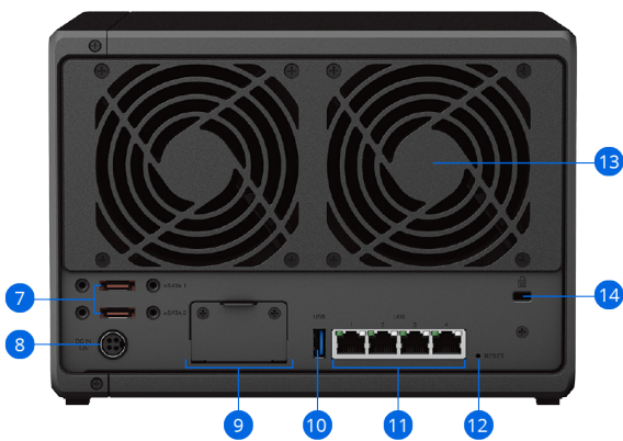
后面板
